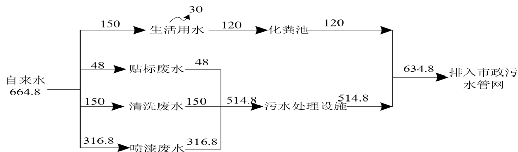
图 2-4 项目用水平衡图 (单位: t/a)
