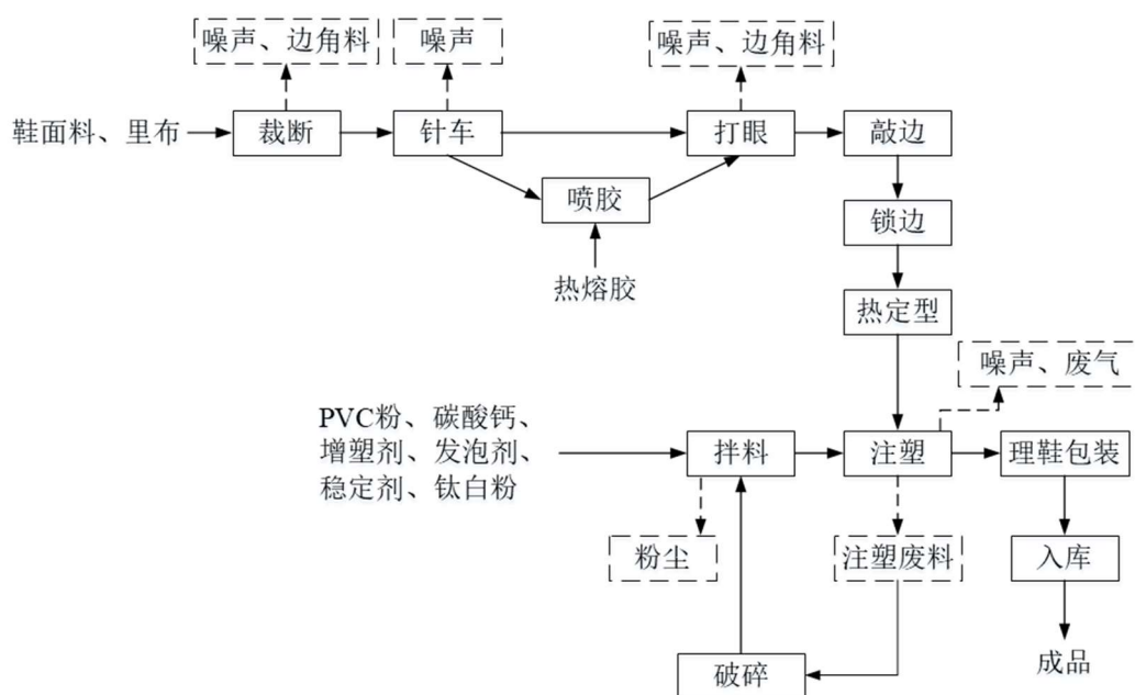
图 2-1 注塑鞋生产工艺流程及产污环节示意图
